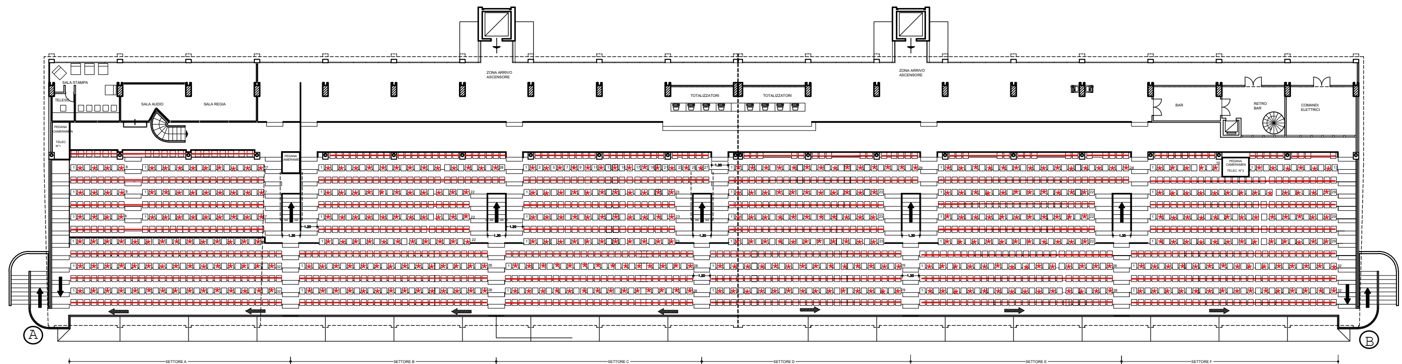
PIANTA PIANO 1° TRIBUNE
